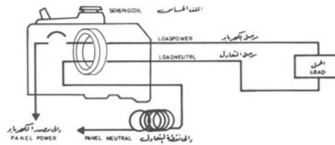
قواطع فوسى مزود بحماية مت تيار التسرب الارضى BRANCH EARTH LEAKAGE CIRCUIT BREAKER
